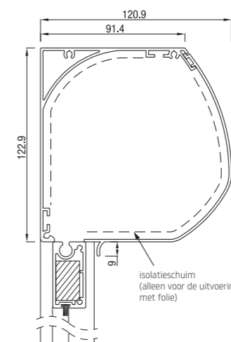
RS Universal 120 dicht
