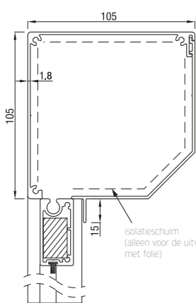
RS Universal 105 schuin
