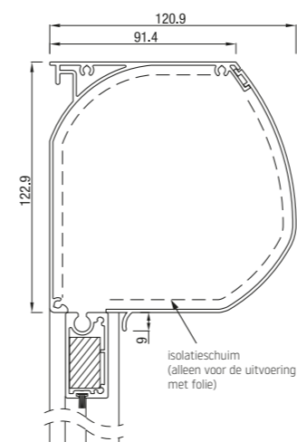
RS Universal 120 half rond
